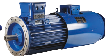
E..DB / E..DC / DD / E..HB / E..HC / HD (Brake) Ex tb IE1-IE2-IE3-IE4 0.18 - 200 kW
